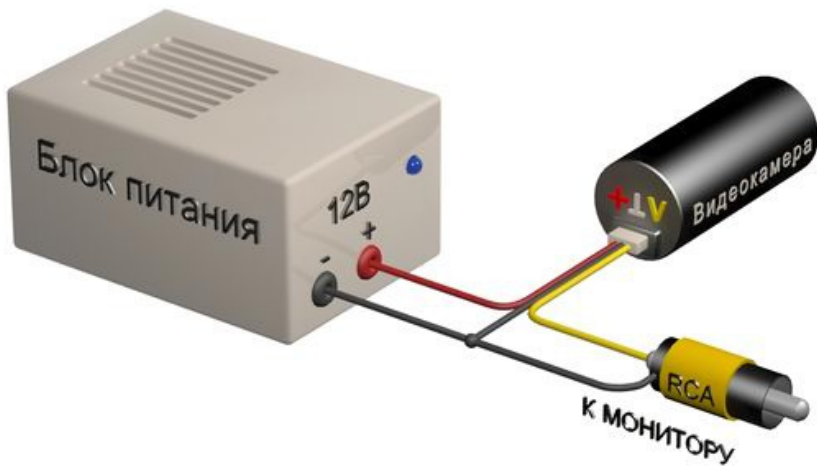
Схема подключения видеокамеры VB19BH-P37C
