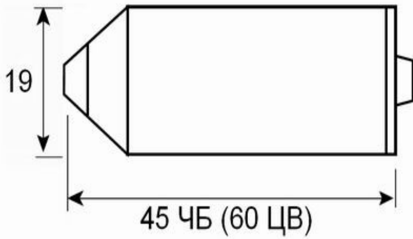
Размеры камеры видеонаблюдения VB19BH-P37C
