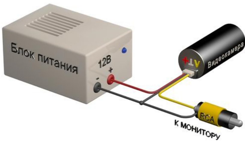
Схема подключения видеокамеры VB19BSHRX-R36
