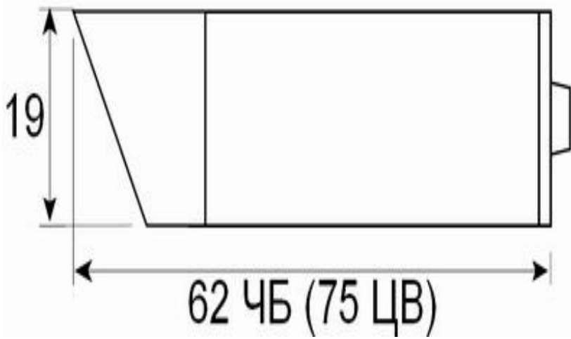
Размеры камеры видеонаблюдения VB19BSHRX-R36
