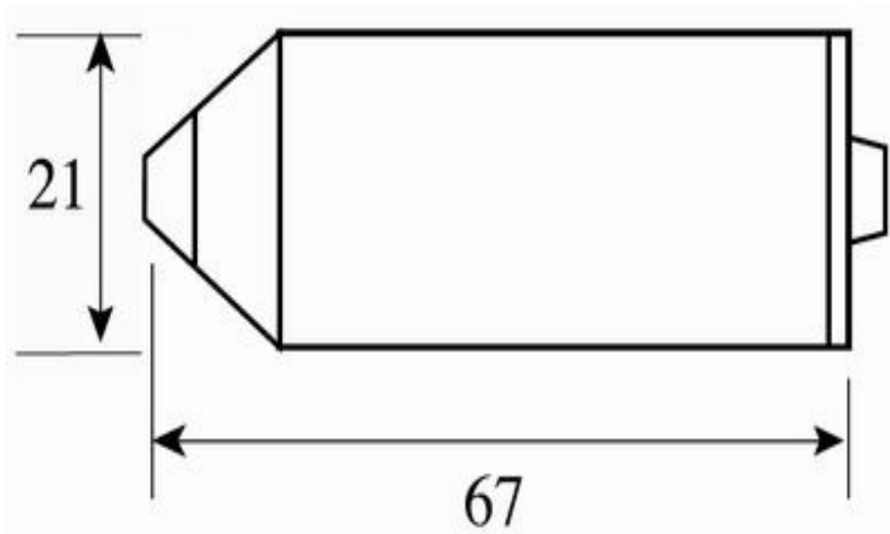
Размеры камеры видеонаблюдения VB21S3-P37C
