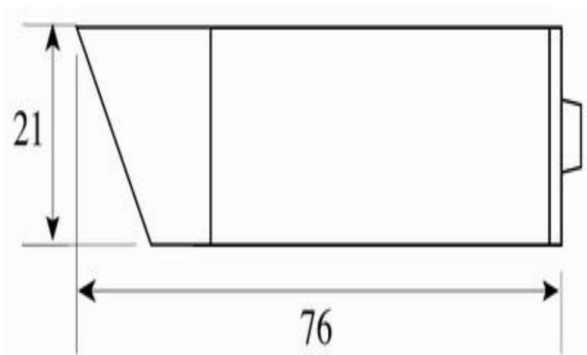
Размеры камеры видеонаблюдения VB21S3-R36
