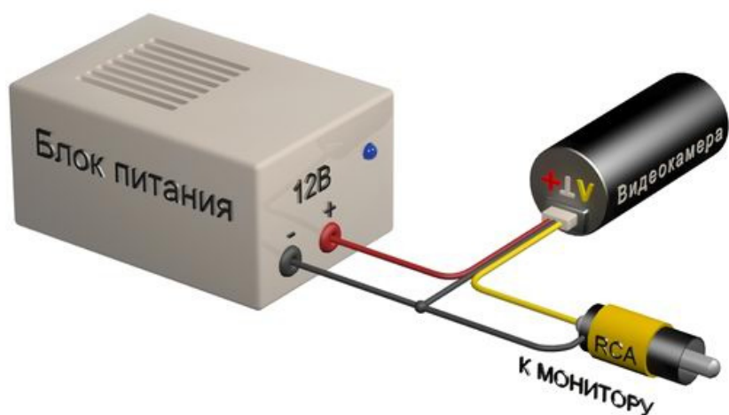
Схема подключения видеокамеры VB21S3-R36
