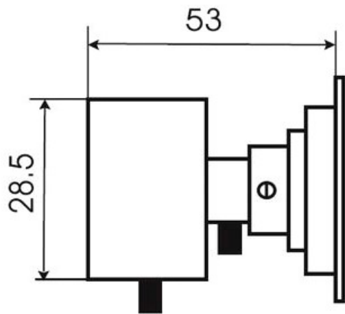
Размеры камеры видеонаблюдения VM32BSHR-VFA49
