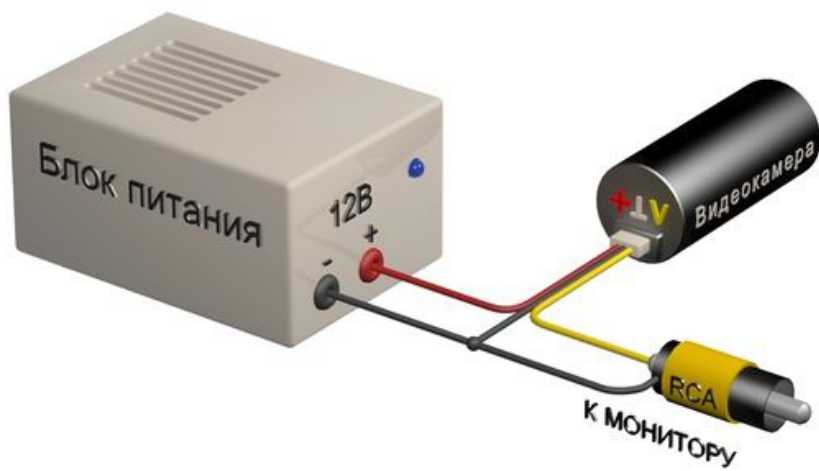
Схема подключения видеокамеры VB19BS-W36
